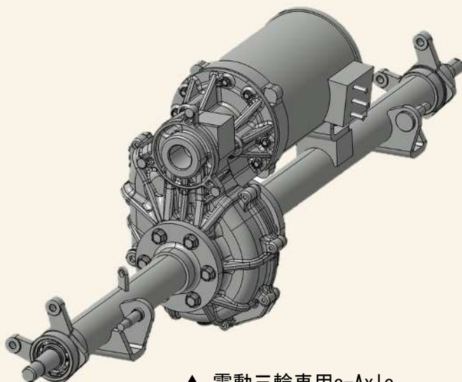
▲ 電動三輪車用e-Axle
