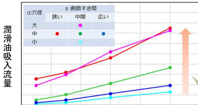
各パラメータと潤滑油吸入流量との関係
